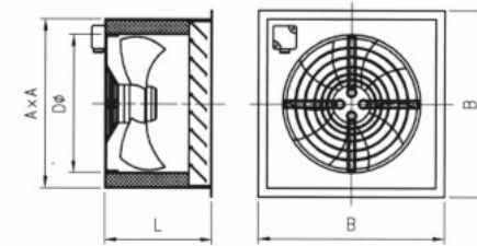
XBDZ 型壁式轴流风机外形及安装尺寸 XBDZ-B 型壁式轴流风机(外转子电机)
