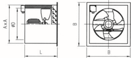
XBDZ 型壁式轴流风机外形及安装尺寸 XBDZ-A 型壁式轴流风机(普通电机)
